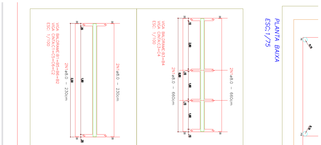
Figura 04 – Projeto estrutural – vigas baldrame e cintas
